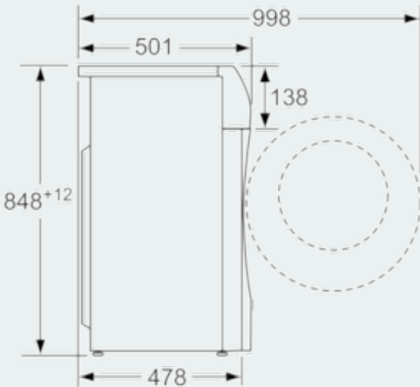
尺寸 (毫米)
