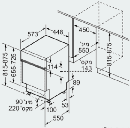
מידות במ"מ
